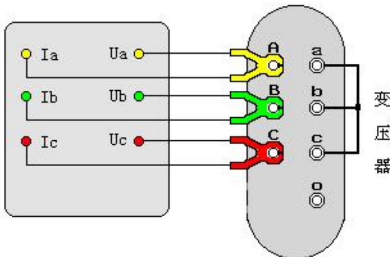
图 24、容量测试接线示意图
